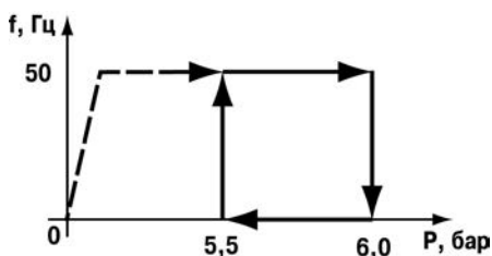
Рисунок 4.17 - Диаграмма алгоритма работы ПЧВ
