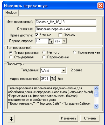
Рисунок 5.13 - Настройка переменной ПЧВ 16-13 Частота, Гц для отображения в OPC
