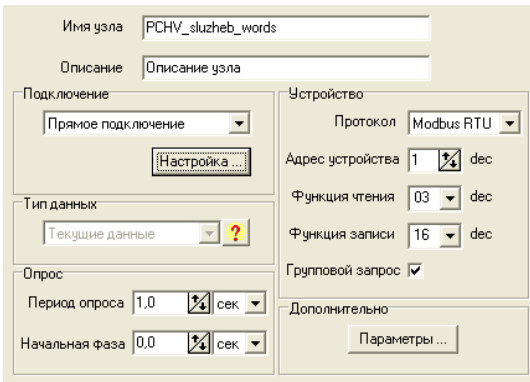
Рисунок 5.12 - Настройки узла PCHV_sluzheb_words
